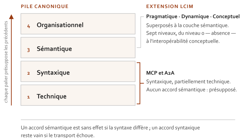
Figure 1.1 — La pile canonique d'interopérabilité, son extension par le LCIM et le palier où opèrent MCP et A2A.
